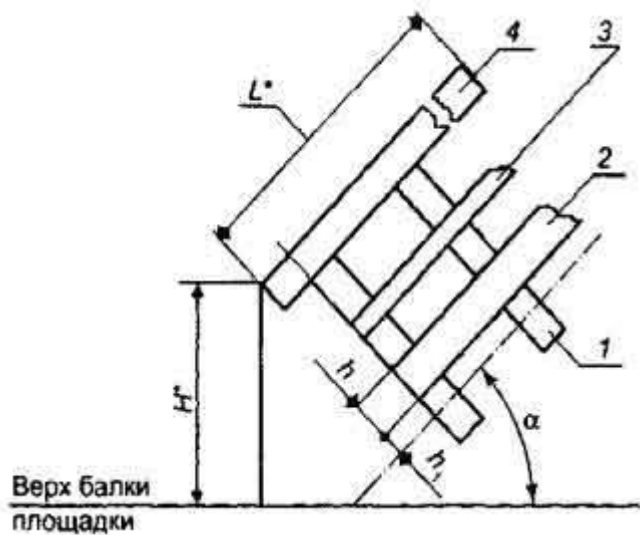
1 - стойка; 2 - бортовой элемент; 3 - средний ограждающий элемент; 4 - поручень
