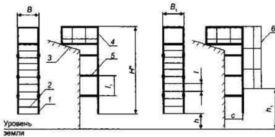
1 - тетива; 2 - ступень; 3 - кровля; 4 - площадка; 5 - балка; 6 - ограждение
