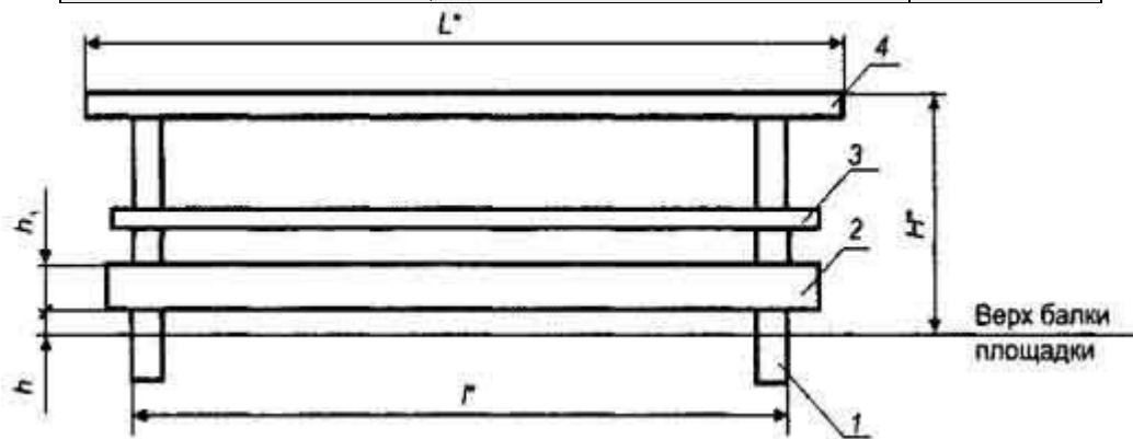
1 - стойка; 2 - бортовой элемент; 3 - средний ограждающий элемент; 4 - поручень
