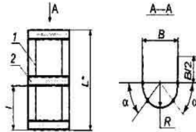
1 - вертикальный ограждающий элемент; 2 - горизонтальный ограждающий элемент
