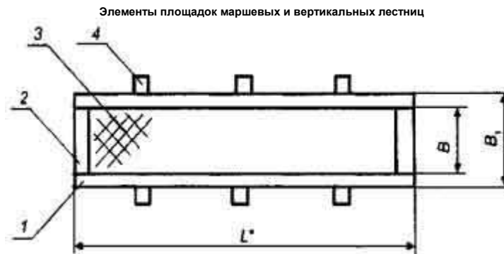
1 - балка; 2 - окантовочный элемент; 3 - настил; 4 - ребро
