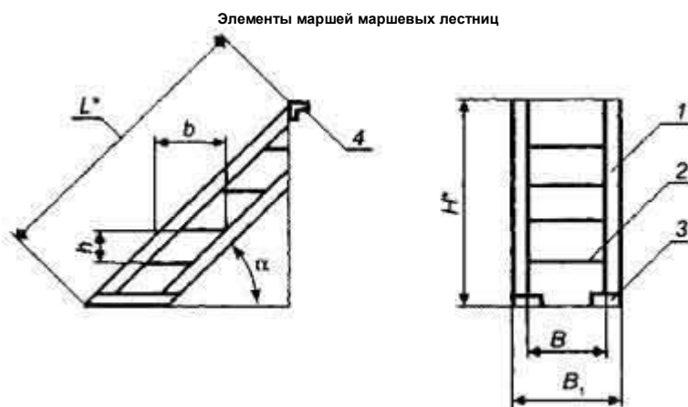
1 - косяур; 2 - ступень; 3 - опорная планка; 4 - опорный уголок
